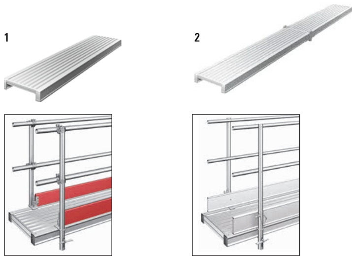
Aufbau mit Geländer-Befestigungsstiel , Gerüstrohren und Normkupplungen.
